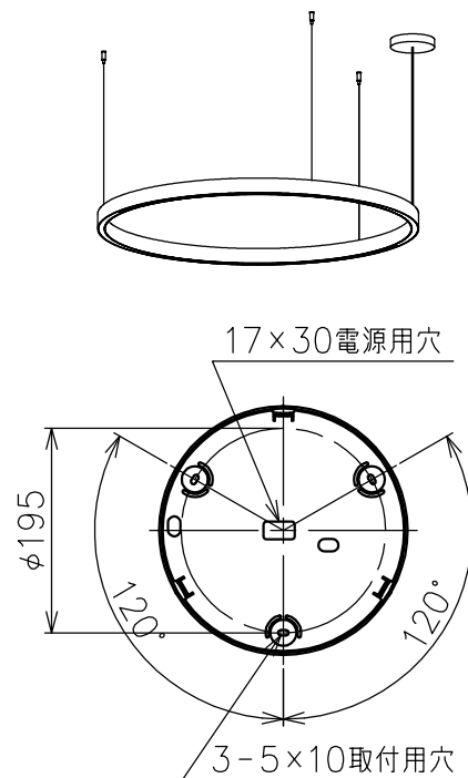
取付板詳細
